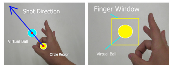
図3. 構え状態の手とおはじきの2点を使った方向の設定(左)と指認識ウインドウの位置(右)。なお本システムでは人差し指や中指を親指にかけて弾く動作を認識対象とする。
