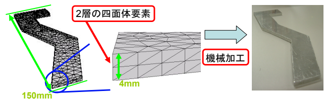
図5. FEMの離散化に用いられたメッシュ。二次元の三角形要素を突き出して作った四面体要素を2段に重ねたものを用いている。
