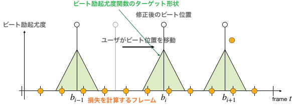
図 5. ユーザ修正から DNN へ与える損失の作成.
