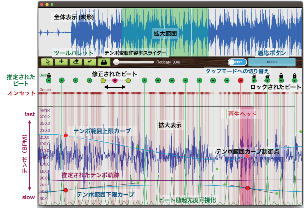
図 2. システム GUI. 楽曲が入力されると波形とともに推定されたビート情報を表示する。システムはユーザに複数種類のビート修正ツールを提供する。
