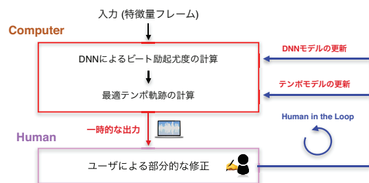
図 1. システム概要。ユーザはシステムの一時的な出力に対して一部分だけを修正してフィードバックする。システムはそれをもとに内部モデルを更新しより所望の結果を出力できるようになっていく。
