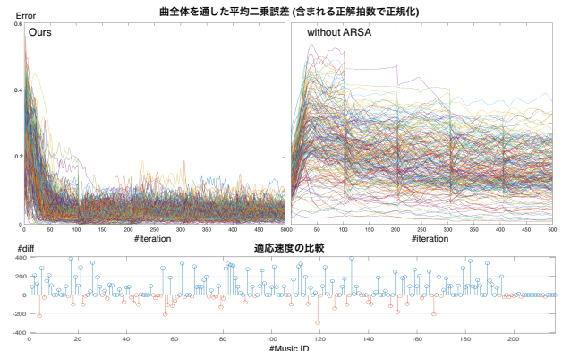
図 7. シミュレーション実験結果。上段：反復回数ともなう各楽曲全体を通した平均二乗誤差の推移。下段：提案手法と比較手法間での収束速度の差分。
