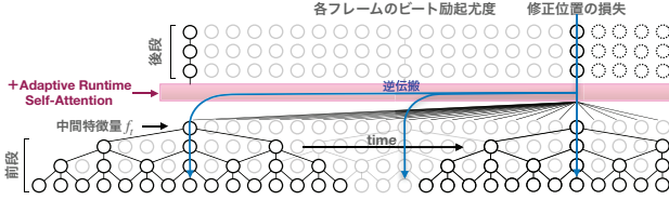
図 6. 実行時には事前学習された DNN を分割し、新たに ARSA ブロックを組み込む.
