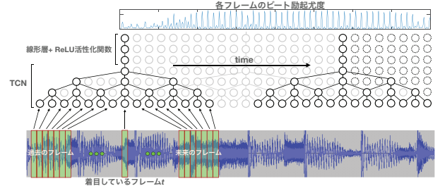
図 4. 事前学習時にはある時刻周辺の局所的な情報を入れてその時刻のビート励起尤度を出力する。
